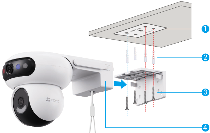
그림 1 천장 장착
