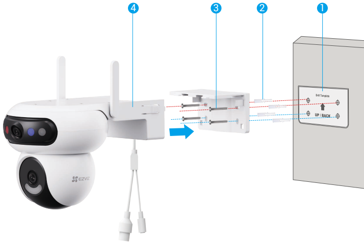
그림 2 벽 장착
